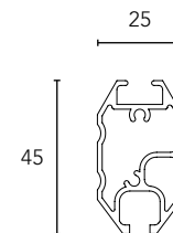
Profilo terminale Terminal bar Profile de barre de charge
